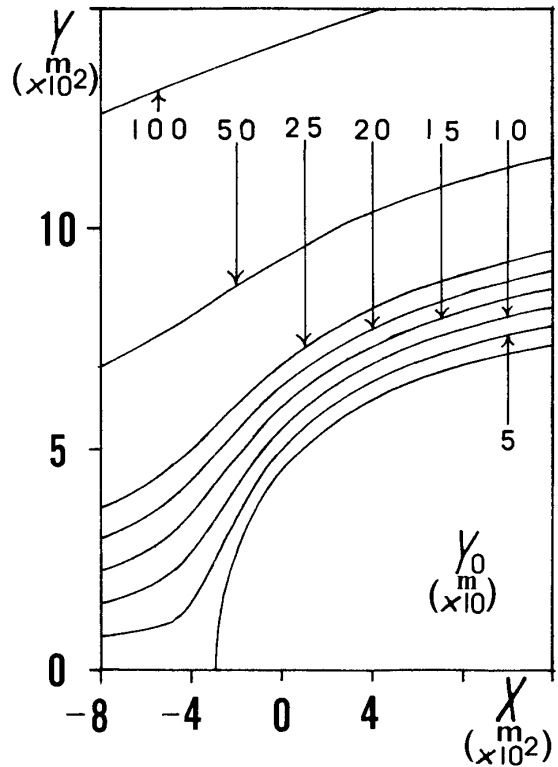
図3 流線 I ( U=6.000\text{ m/s} , b=9.000 \times 10^2\text{ m} )
