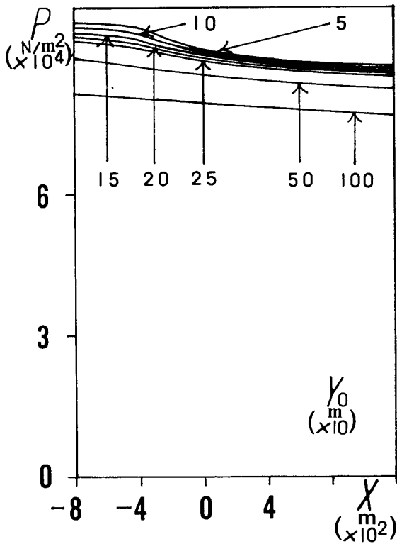
図4 気圧 ( U=6.000\text{ m/s} , b=9.000 \times 10^2\text{ m} )
