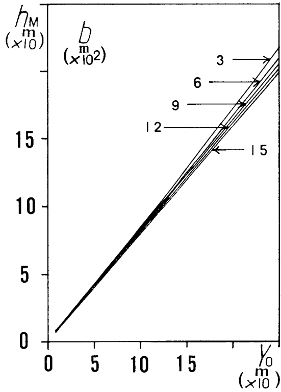
図5 山の面から一つの流線上での最大風速点までの高さ ( U=6.000\text{ m/s} )
