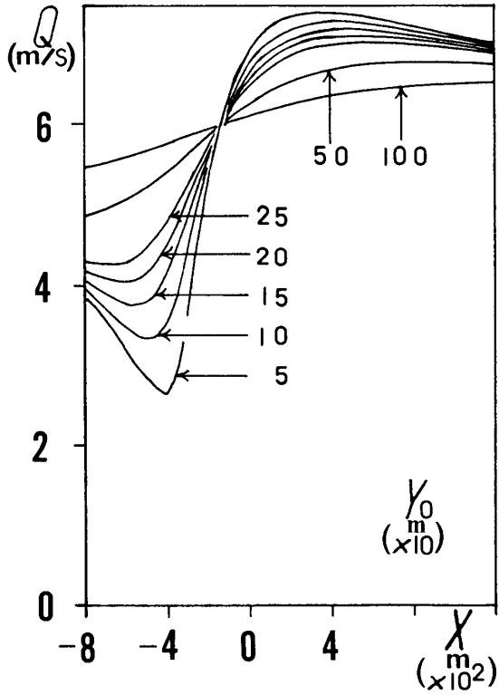
図2 風速 I ( U=6.000\text{ m/s} , b=9.000 \times 10^2\text{ m} )
