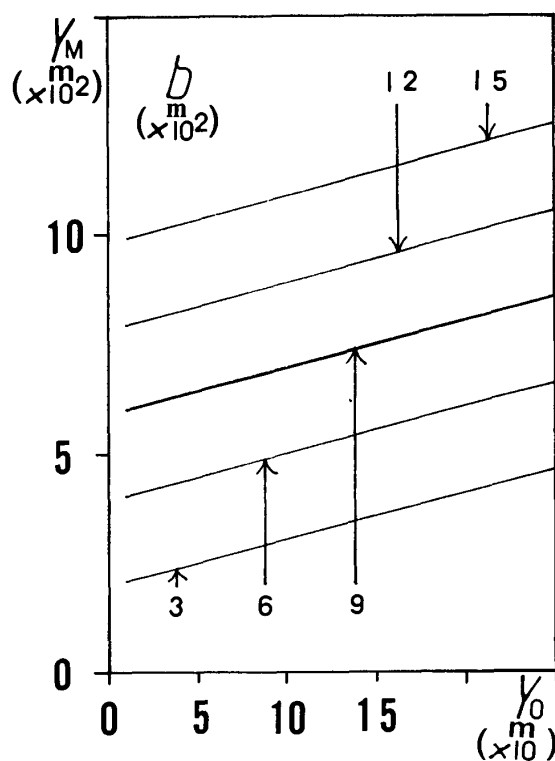
図7 一つの流線上での最大風速点のY座標 ( U=6.000\text{ m/s} )
