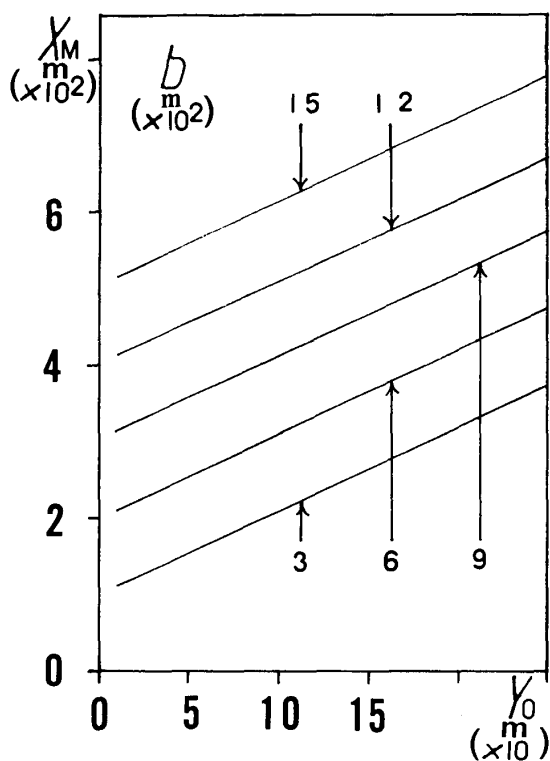
図6 一つの流線上での最大風速点のX座標 ( U=6.000\text{ m/s} )
