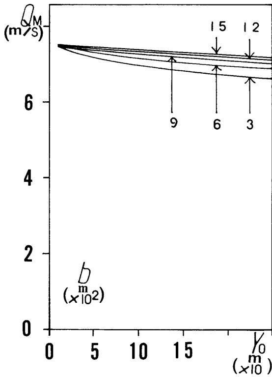
図8 一つの流線上での最大風速 ( U = 6.000 \text{ m/s} )
